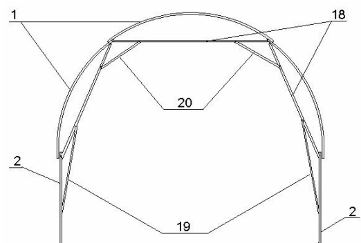
Рис.5 Усилитель арки
